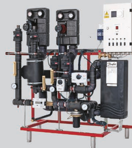
Red Frame Type DSP 1, MIDI Gulvstillet urt til varme - med svejste rør og loddet pladevarmeveksler
